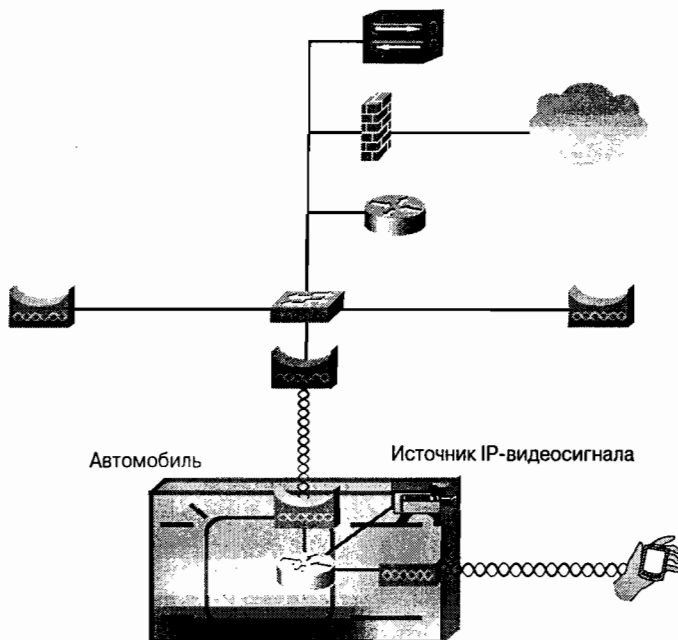
Рис. 10.7. Пример сети в сфере общественной безопасности
