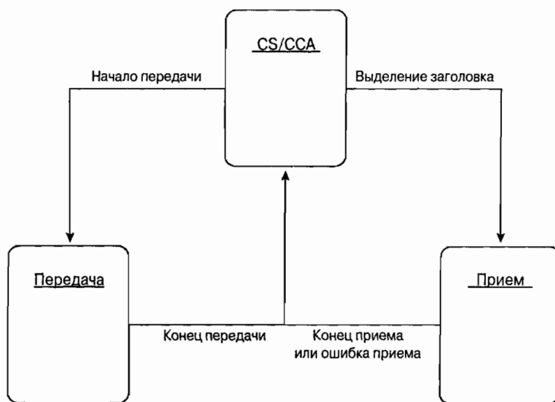
Рис. 3.2. Диаграмма состояний PLCP
