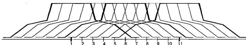
Рис. 7.9. Неперекрывающиеся каналы стандарта 802.11b
