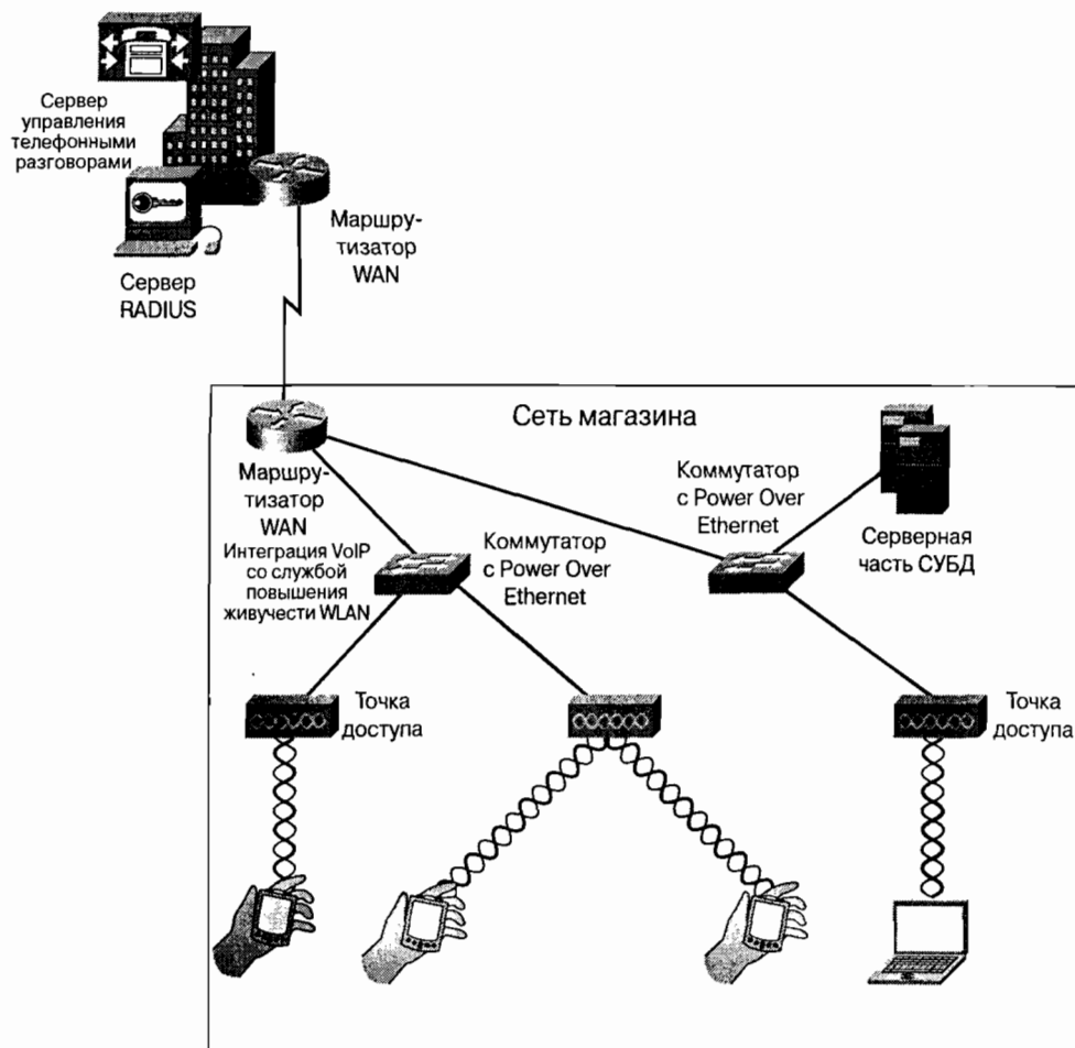
Рис. 10.2. Сеть магазина розничной торговли с механизмами повышения живучести
