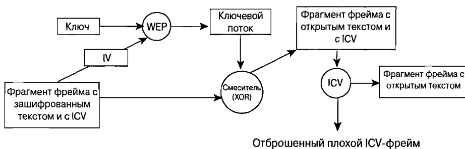
Рис. 4.7. Процесс шифрования и дешифрования
