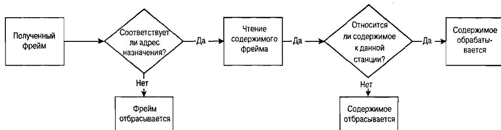
Рис. 1.6. Станция определяет, должна ли она обрабатывать фрейм
