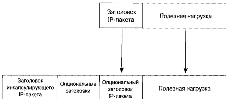
Рис. 5.14. Инкапсуляция IP-пакетов
